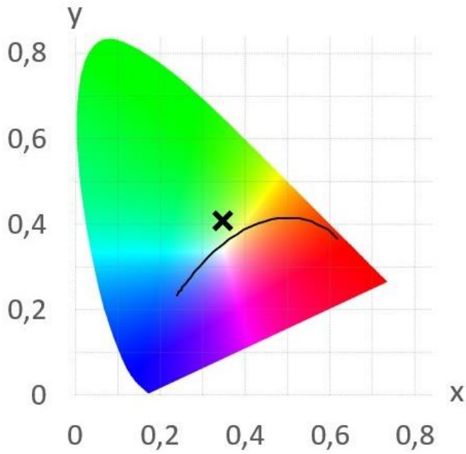
CIE1931 UV:
